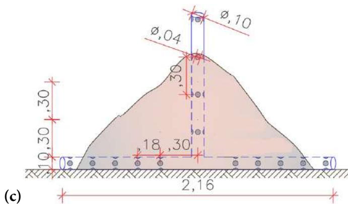
Figura 5 – Detalhe da montagem das pilhas de compostagem naturalmente aerada utilizando tubo T perfurado (a) e vista das pilhas formadas (b). Experimento piloto conduzido durante vigência do INCT ETEs Sustentáveis (c e d) (medidas expressas em metros).
