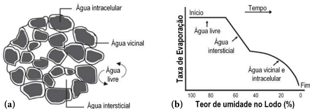
Figura 1 – (a) Forças de ligação da água presente no lodo; (b) Curva típica de secagem de lodo.
