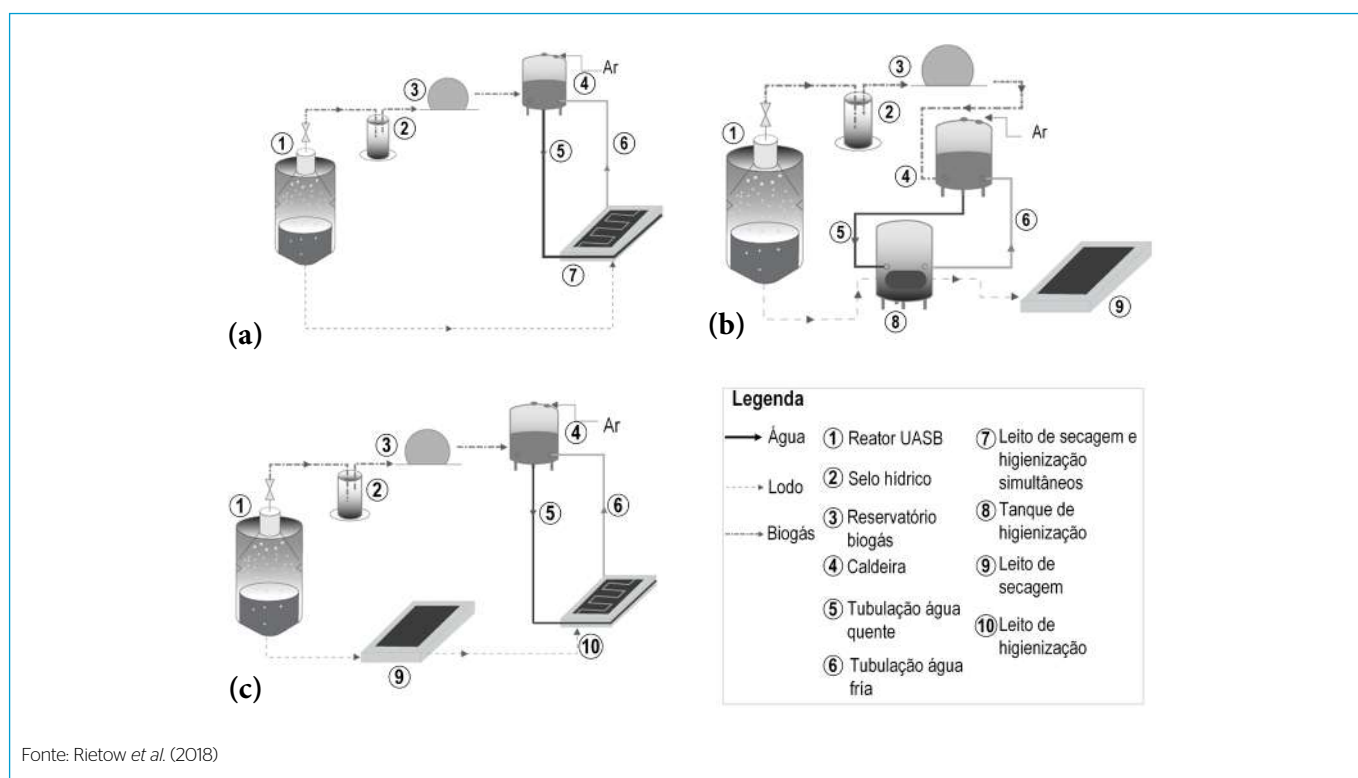
Figura 5 – Sistemas simplificados de secagem e higienização térmica do lodo para ETES de pequeno e médio porte: (a) leito de secagem convencional modificado para promover a secagem e higienização do lodo de forma simultânea; (b) tanque aquecido para higienização seguido de leito de secagem convencional; (c) leito de secagem convencional seguido de leito aquecido para higienização.
