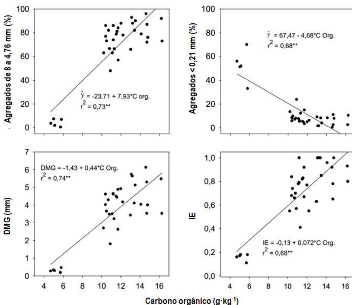
Figura 2 - Relação entre teor de carbono orgânico do solo e: (a) agregados da classe de 8,00 a 4,76 mm; (b) agregados menores que 0,21 mm; (c) diâmetro médio geométrico padrão (DMG); (d) índice de estabilidade de agregados (IE).
