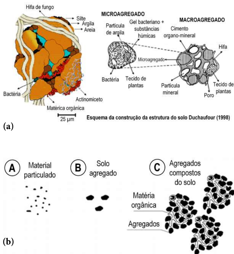
Figura 1 - (a) Modelo de estruturação do solo e o papel da matéria orgânica; (b) esquema ilustrando a formação de agregados do solo a partir de partículas unitárias: A. partículas unitárias do solo (areia, silte e argila), B. microagregados, C. conjunto de macroagregados em solo
