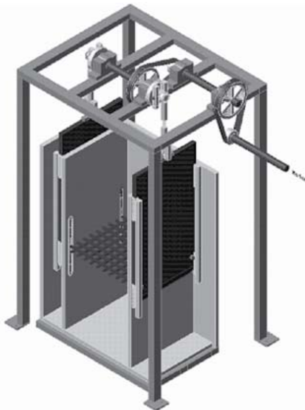
Figura 1 - Tanque de grade oscilante, com seção transversal quadrada de 50,0 cm x 50,0 cm e altura de 115,0 cm. Para a visualização da grade, foram removidas do desenho duas placas de acrílico externas
