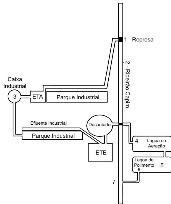
Figura 1 - Esquema ilustrativo dos pontos de coleta e seqüência da captação, utilização e descarte da água utilizada pela empresa de papéis reciclados, Governador Valadares - MG
