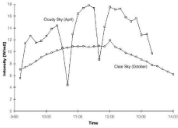
Figura 8 - Variação diária da intensidade de radiação solar UV-A em duas épocas diferentes do ano na região de Beirute - Líbano (SODIS, 2003)
