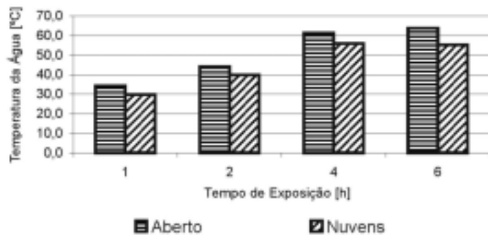
Figura 11 - Temperatura média da água durante o processo de desinfecção solar
