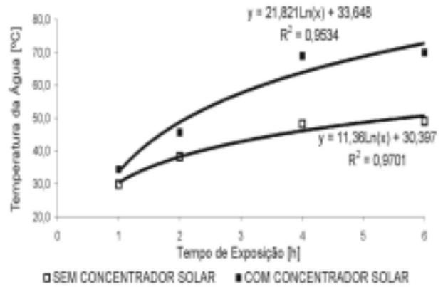
Figura 9 - Temperatura média da água no processo de desinfecção solar (SODIS)
